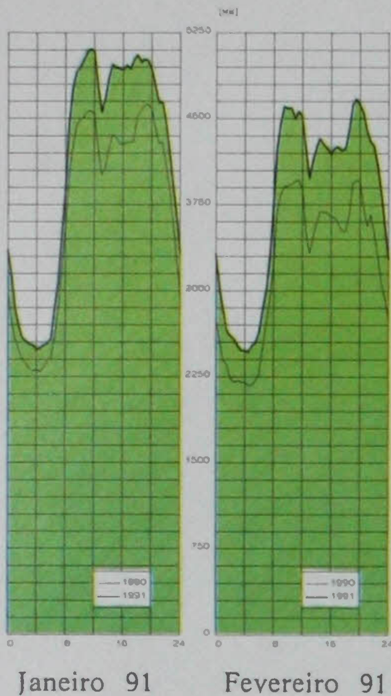
Fig. 1 — Diagramas de consumo das terceiras 4.ª feiras, referido à produção sem bombagem, em 1991 (traço grosso) e 1990 (traço fino), nos meses de Janeiro (à esquerda) e de Fevereiro (à direita)
