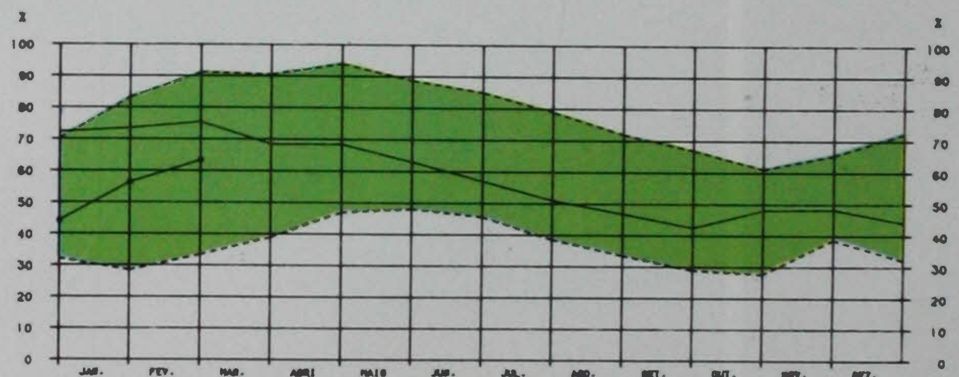
Fig. 4 — Evolução do armazenamento no conjunto das albufeiras, no final do mês, com 100 % correspondente a 2326 GWh, em 1990 (traço cheio) e 1991 (traço com pontos). Traço-traço superior: envolvente de máximos de 1980 a 1989; traço-traço inferior: envolvente de mínimos 1980 a 1989
